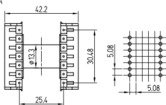
Ansicht A view A
