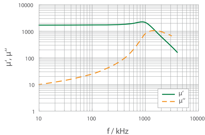
Permeabilität \mu als Funktion der Frequenz f Permeability \mu vs. frequency f
