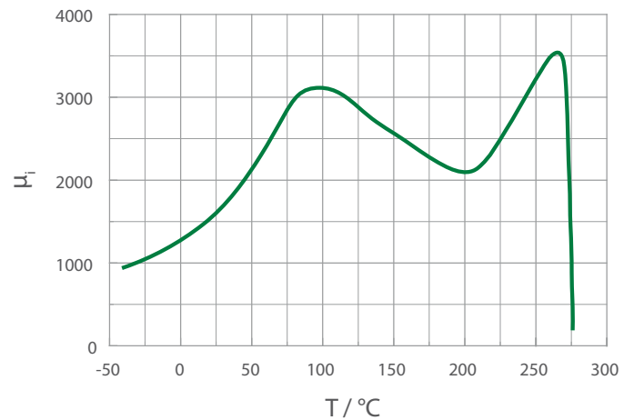
Anfangspermeabilität \mu_i als Funktion der Temperatur T Initial permeability \mu_i vs. temperature T
