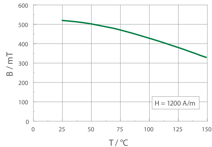
Flussdichte B als Funktion der Temperatur T Flux density B vs. temperature T
