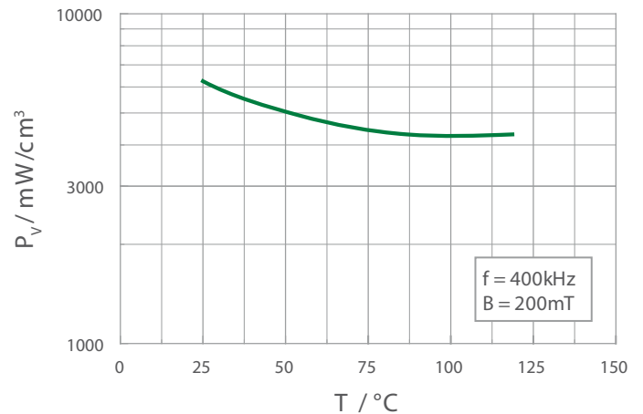
Spez. Verluste P_V als Funktion der Temperatur T Spec. losses P_V vs. temperature T
